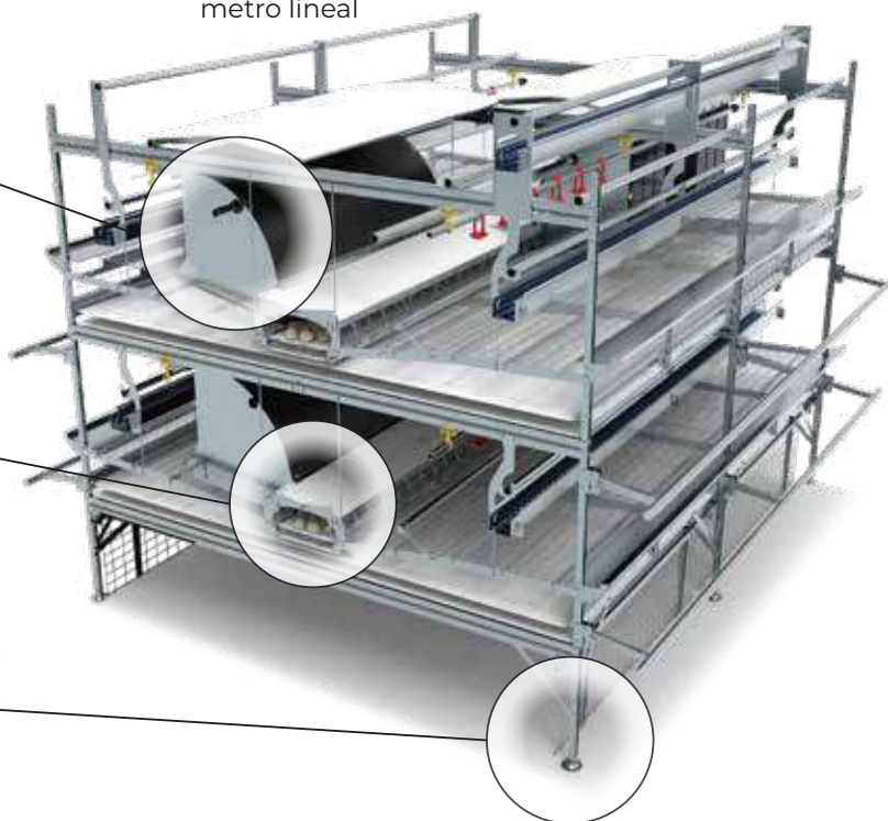
Cinta central de huevos en cada hilera de 290 mm de ancho
