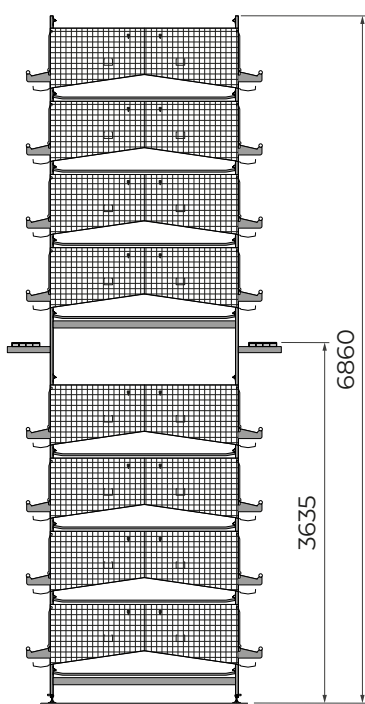
8 étages DD
