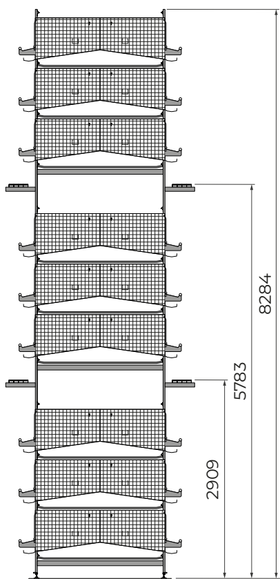
9 étages TD
