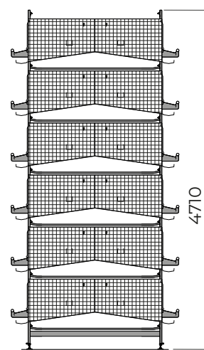
6 étages
