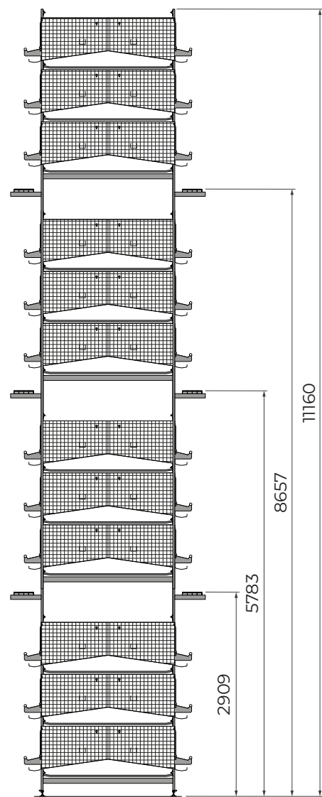
12 étages QD
