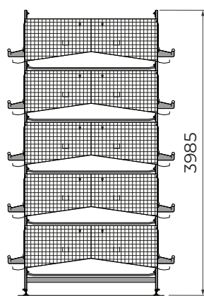
5 étages
